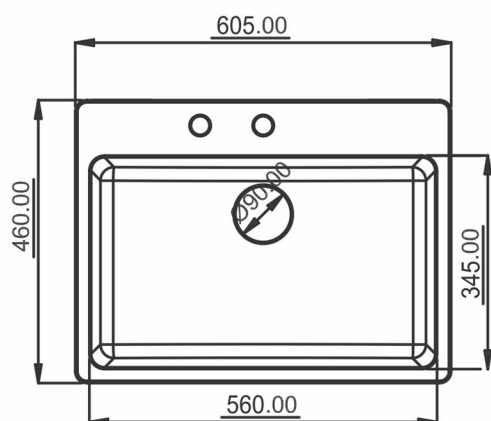
DIMENSIONS
